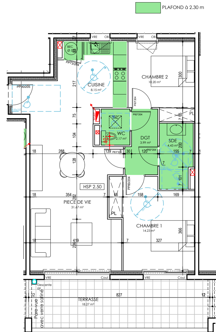
• Plan 1 / 100
