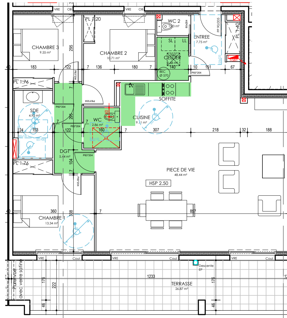
• Plan 1 / 100
