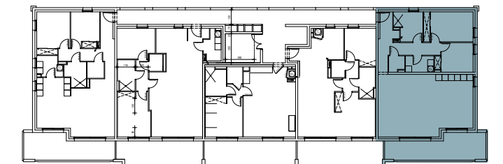
• Plan R+2
