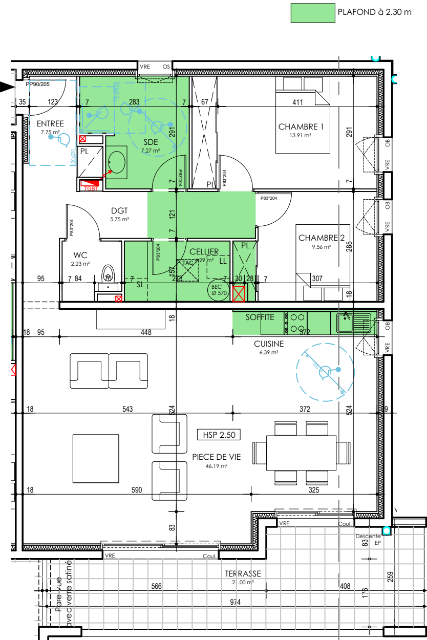
• Plan 1 / 100
