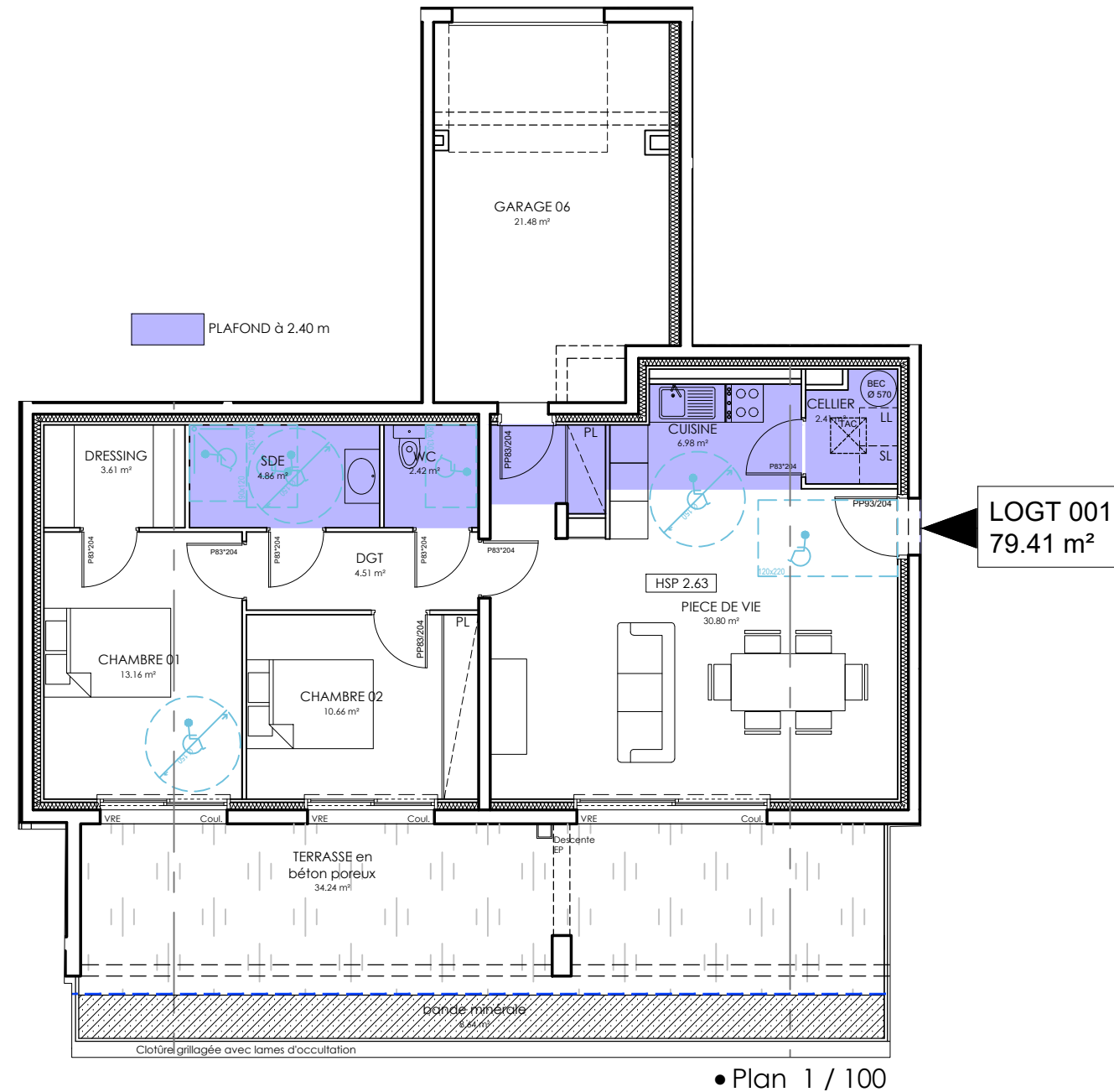
• Plan Rez de Chaussée
