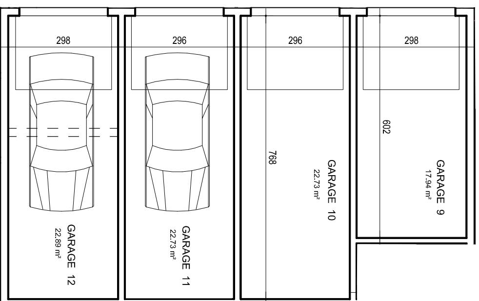
• Plan 1 / 100
